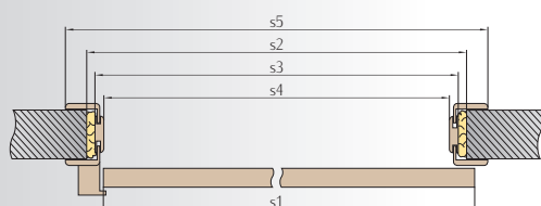
SYSTÉM MONTOVANÝ ZA POUŽITÍ REGULOVATELNÉHO TUNELU
