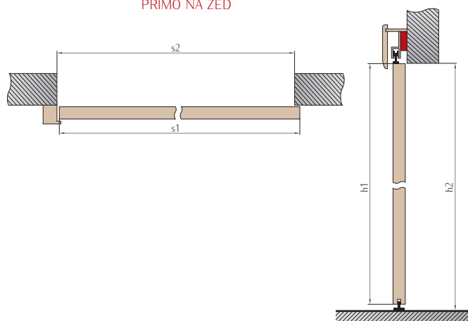
SYSTÉM MONTOVANÝ PŘÍMO NA ZEĎ
