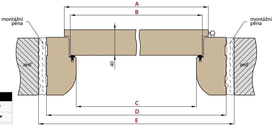
■ NÁKRES RÁMOVÉ ZÁRUBNĚ
